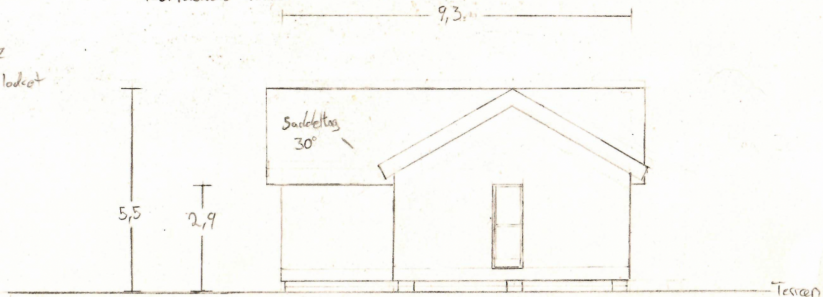
Vestfacade 1:100
